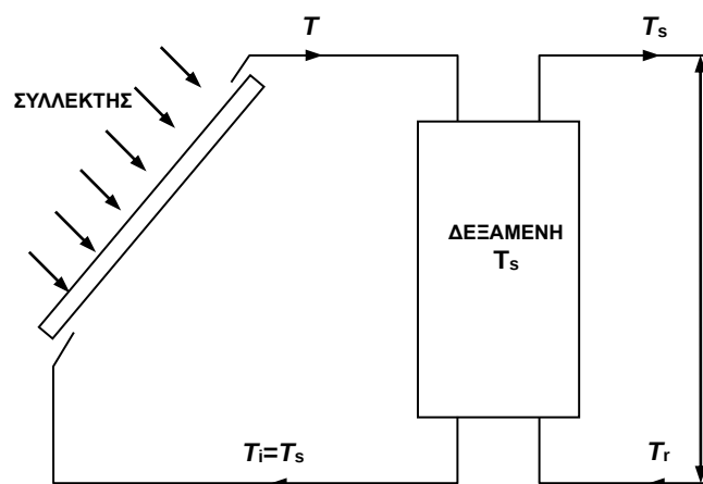
Σχήμα 6.1: Ηλιακό σύστημα θερμού ύδατος (Πηγή: Γιαννοπουλος, 2005)
